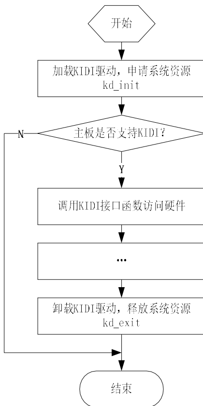
图 5.2 KIDI 驱动接口调用流程图
